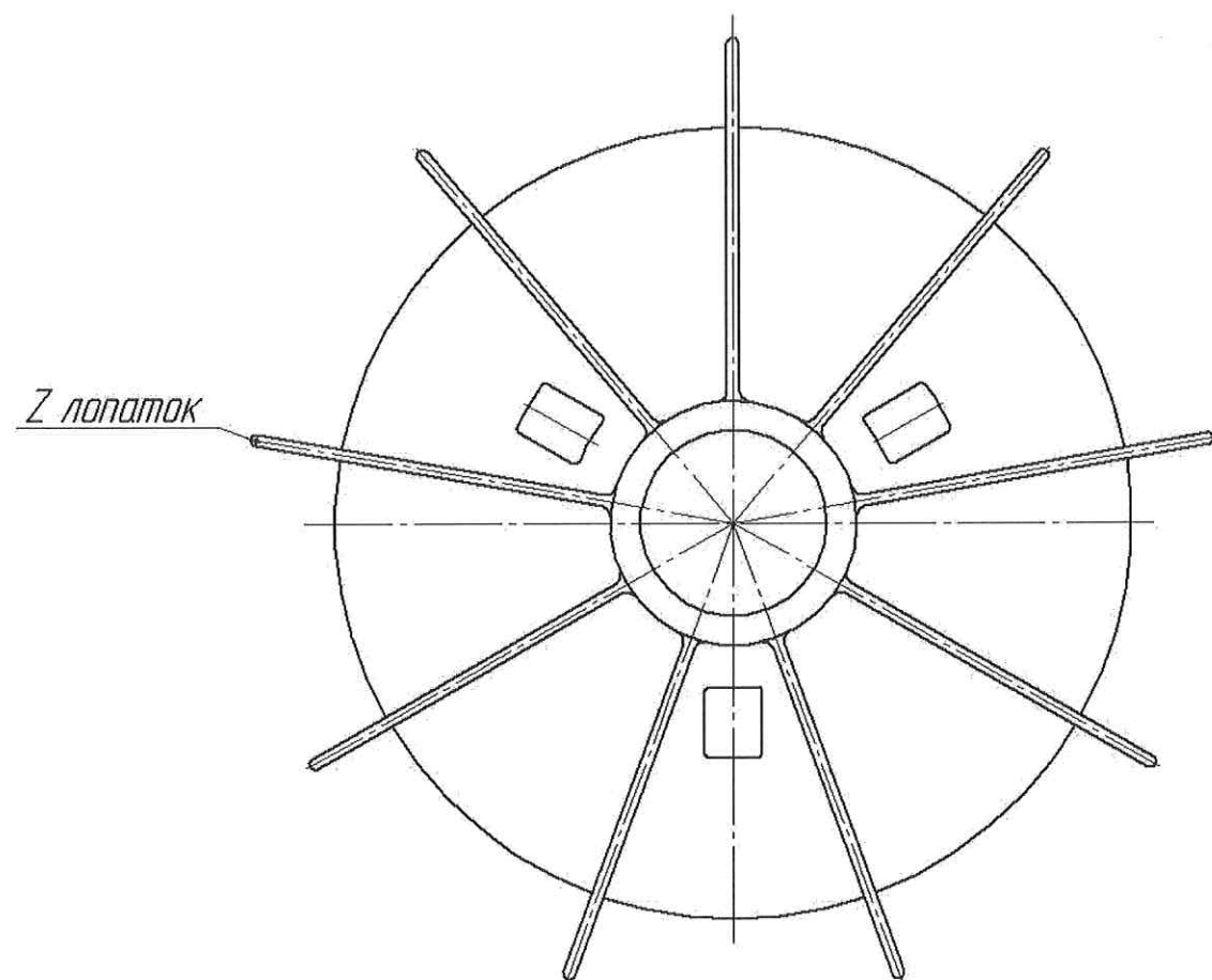
Чертеж крыльчатки
